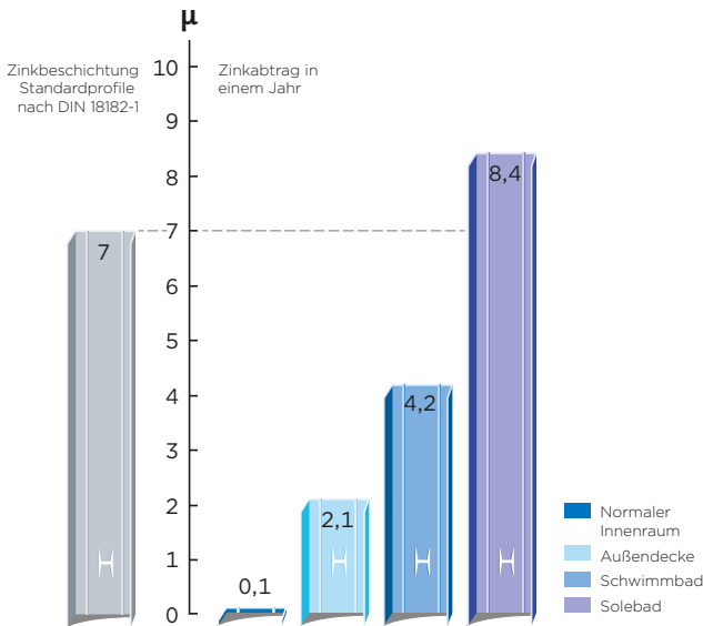
Atmosphärische Korrosivität, Zinkabtrag nach EN ISO 9224:2012
