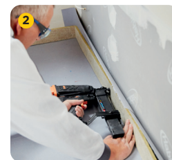
Randdämmstreifen verlegen
