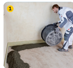
Schüttungsmaterial ausbringen
