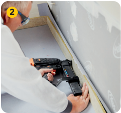
Randdämmstreifen verlegen
