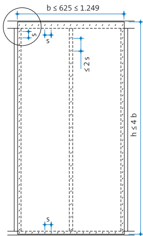
Einraster-Tafel, Befestigung der 1. Lage mit Stahldrahtklammern
