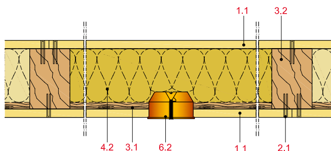
Einbau einer EIt.-Dose mit Steinwolle
