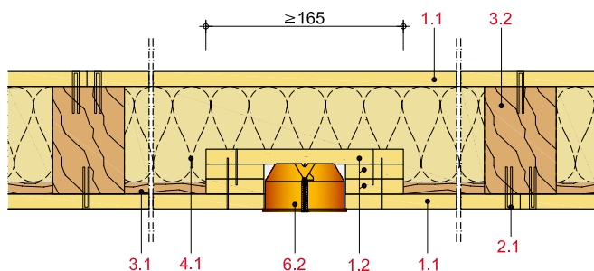
Einbau einer EIt.-Dose mit Einhausung
