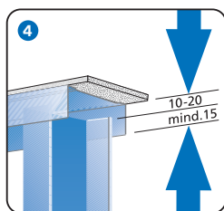
Abfangung zusätzlicher Auflagerkräfte
