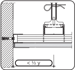
y = Abstand Grundprofil
