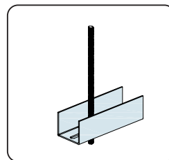
Gewindestangen \geq M8 (Steg unterseitig)
