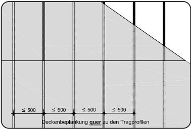
Deckenbeplankung quer zu den Tragprofilen
