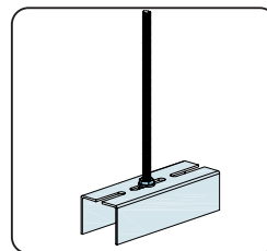
Gewindestangen \geq M8 (Steg oberseitig)
