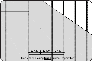
Deckenbeplankung längs zu den Tragprofilen
