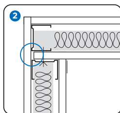
Wandecke mit CW-Ständern als Alternative
