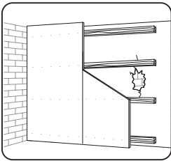
Vorsatzschale auf Holzlattung
