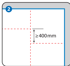
Horizontalfugen bei 1-lagiger Beplankung
