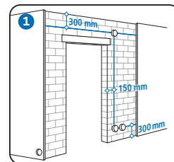
Alle Unterputz-Installationen sind vorher abzuschließen
