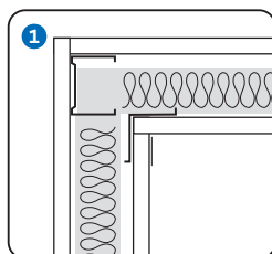
Wandecke mit Rigips Wandprofil LWI, die einfachste und schalltechnisch günstigste Ausführung
