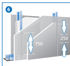
Schraubenabstände für Montagewände mit Doppelbeplankungen
