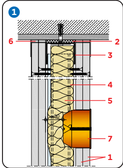
Einbau der Elektrodose in Montagewand mit gestauchter Mineralwolle ≥ 30 kg/m³, Schmelzpunkt ≥ +1.000 °C (Rigips Detail MW12-D-ED-1)
