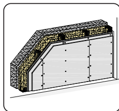
Vorsatzschale freistehend
