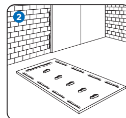
Aufbringen des Rifix Ansetzbinders
