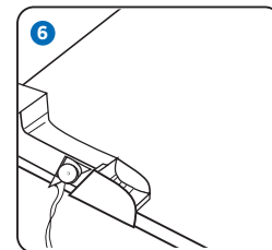
Schnittkanten mit VARIO Kantenhobel anfasen
