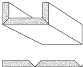
2 x V-Fräsung 90° von der Rückseite
