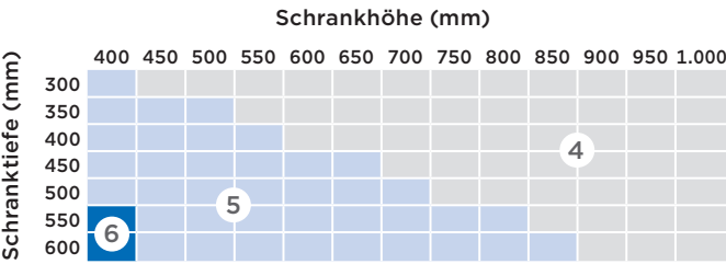
Anzahl notwendiger Grobgewindeschrauben
