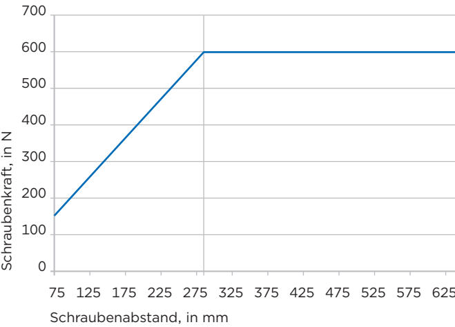
Zulässige Schrauben- und Traversenbelastung in Abhängigkeit des Schraubenabstandes
