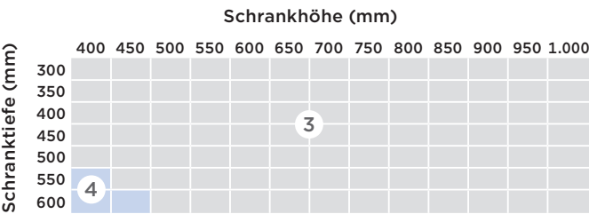
Anzahl notwendiger Metallhohlraumdübel
