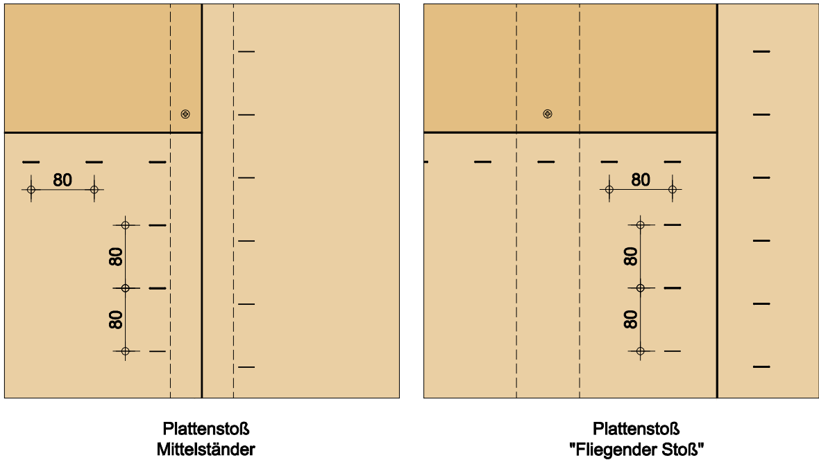
Abbildung 8: Verklammerung „Die Harte“ auf „Die Harte“ Detail 2
