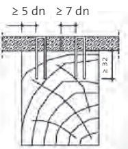
Klammernbefestigung Stoß
