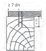
Klammernbefestigung Tafelränder
