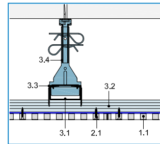
Stirkantenstoß Rigitone
