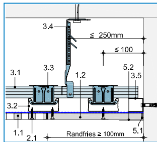
Längsseite
