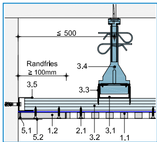
Querseite
