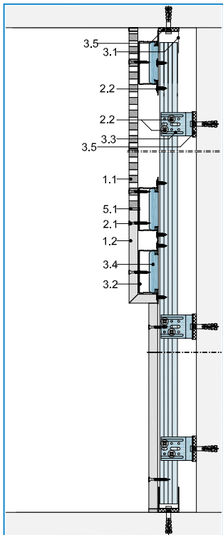
Variante 2 Vorsatzschale mit Unterkonstruktion und Absorberelement im oberen Wandbereich
