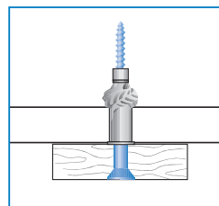
Expandier-Dübel
