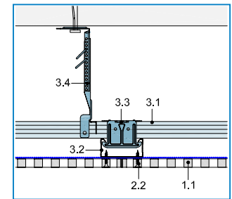
Längskantenstoß Rigitone
