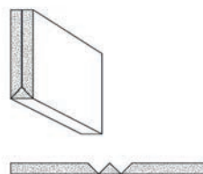
2 x V-Fräsung 90° von der Rückseite
