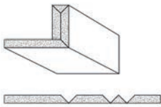
3 x V-Fräsung 90° von der Rückseite
